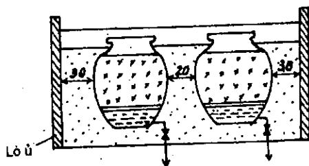
14a) Ang sành trích ly
