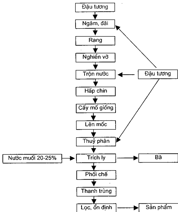
Hình 9: Quy trình kỹ thuật sản xuất nước chấm lên men từ đậu tương
