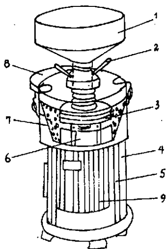
Hình 2: Cấu tạo máy xay bột nước Trung Quốc
