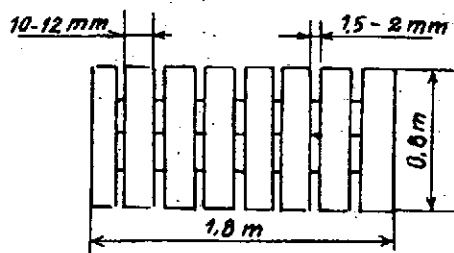
a) Mảnh tre để nuôi mốc
