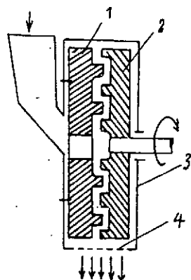
Hình 7a: Máy nghiền loại đĩa răng
