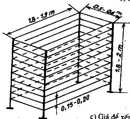
c) Giá để xếp mảnh mốc
