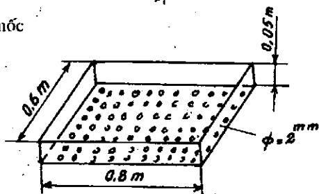
b) khay nhôm để nuôi mốc.
