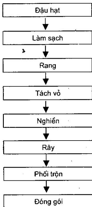
Hình 6: Sơ đồ công nghệ sản xuất bột đậu tương
