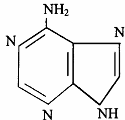
Gốc purin
