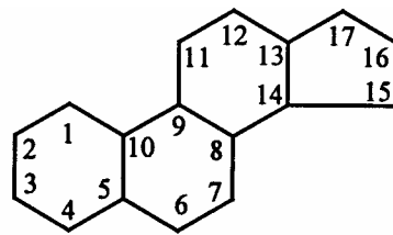
Nhân cyclopentanhydrophenantren
