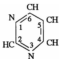
Gốc pyrimidin
